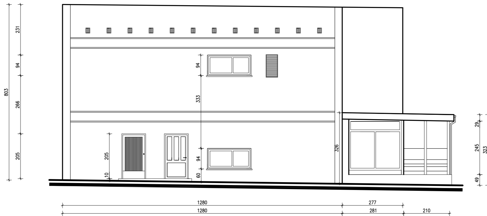
ELEWACJA WSCHODNIA
